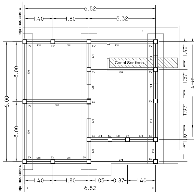
PLANTA DE LOSAS
