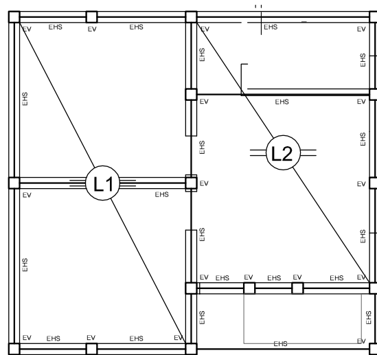
PLANTA DE LOSAS
