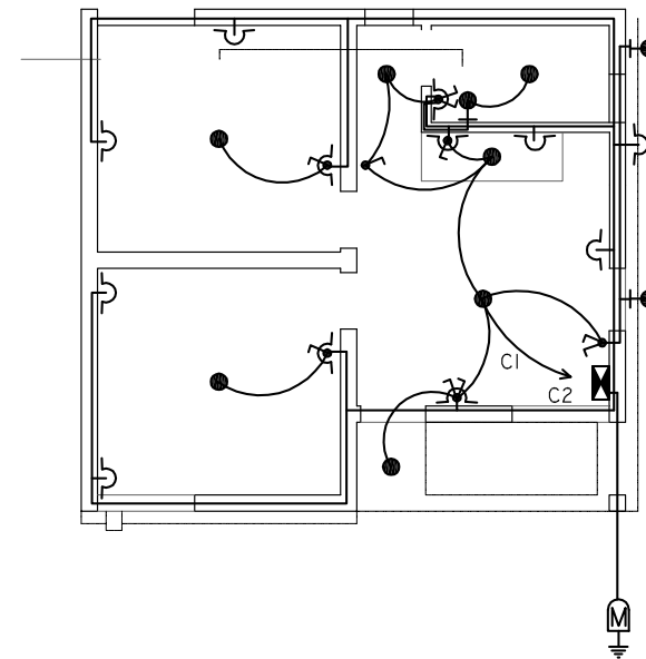
PLANTA DE ELECTRICIDAD
